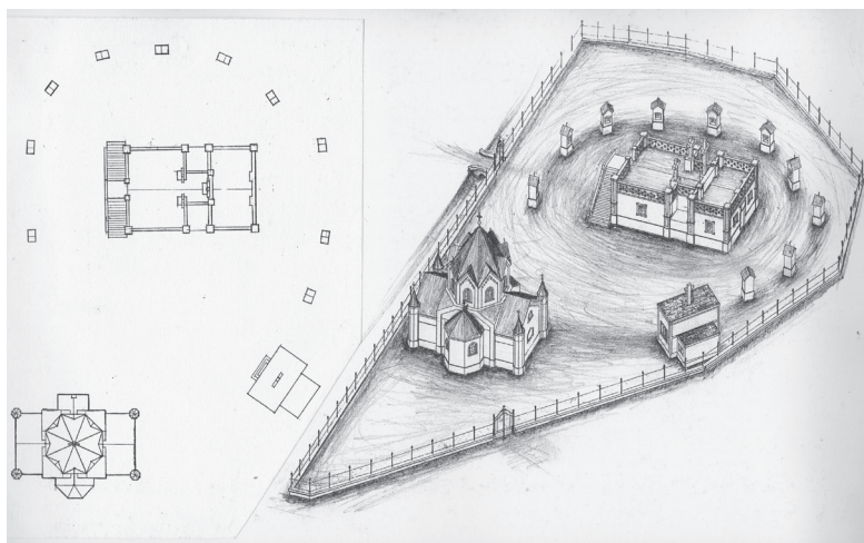
Axonometrikus rekonstrukciós rajz és alaprajz a Rónay-sírketről
