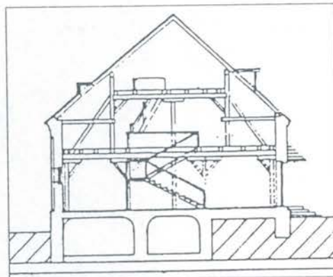
A magtár metszete
